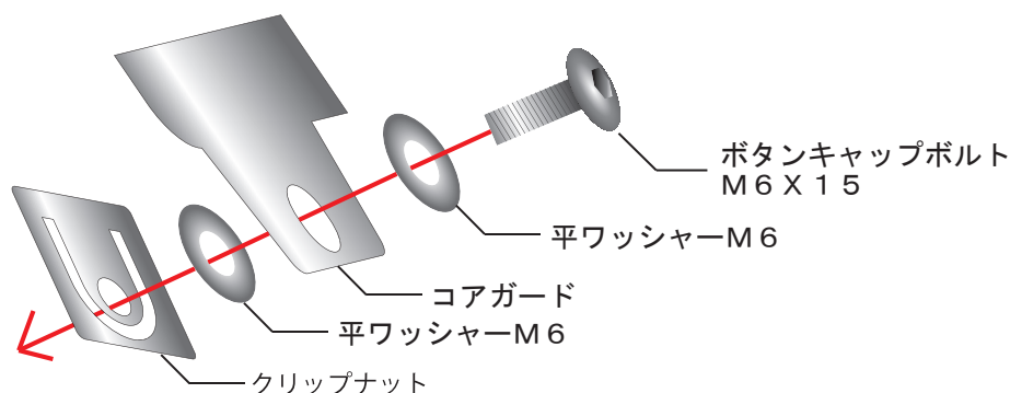
図1 ラジエター本体ステーに下から差し込む
