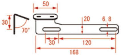
寸法図
